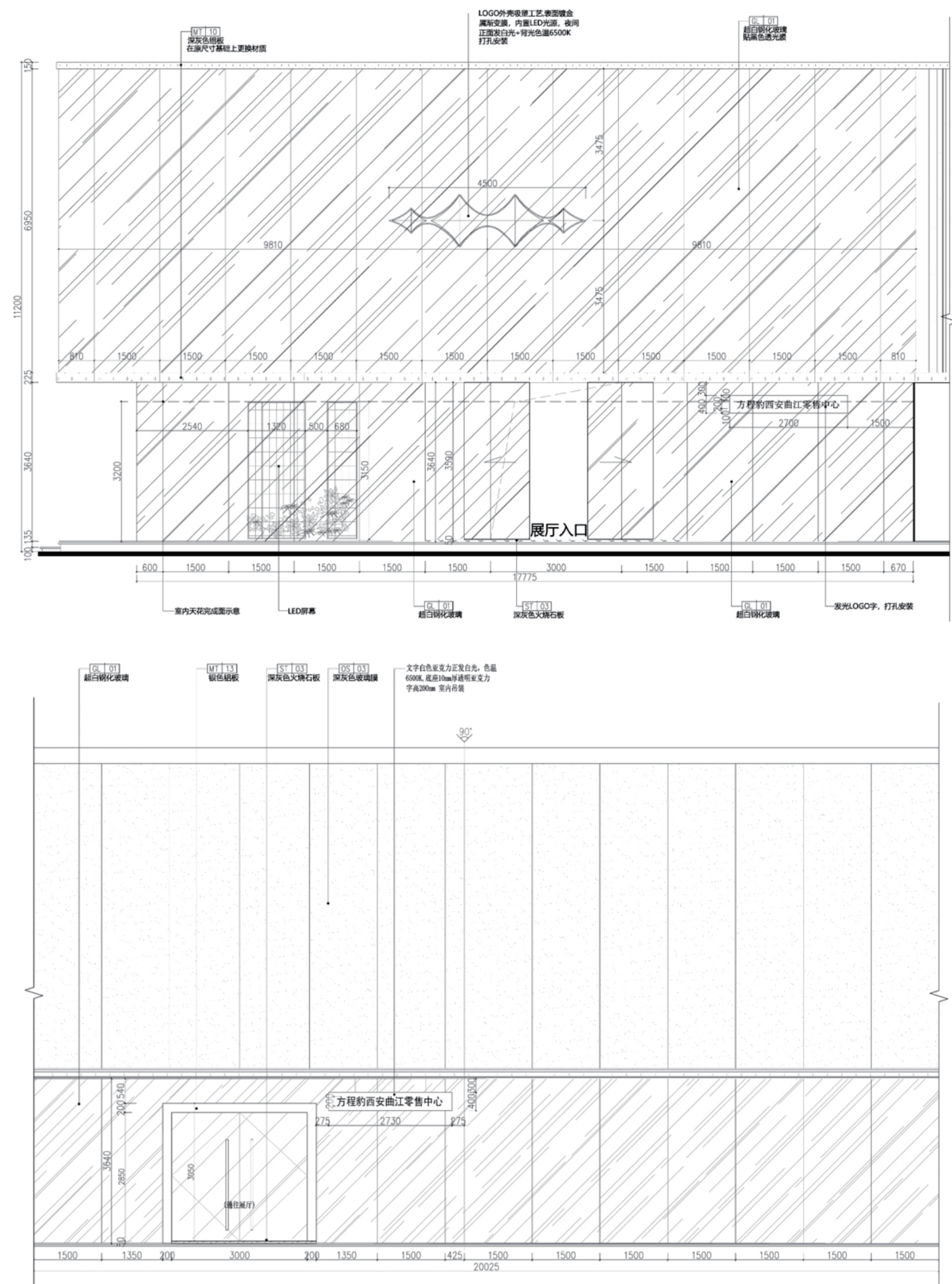
外立面示意图
