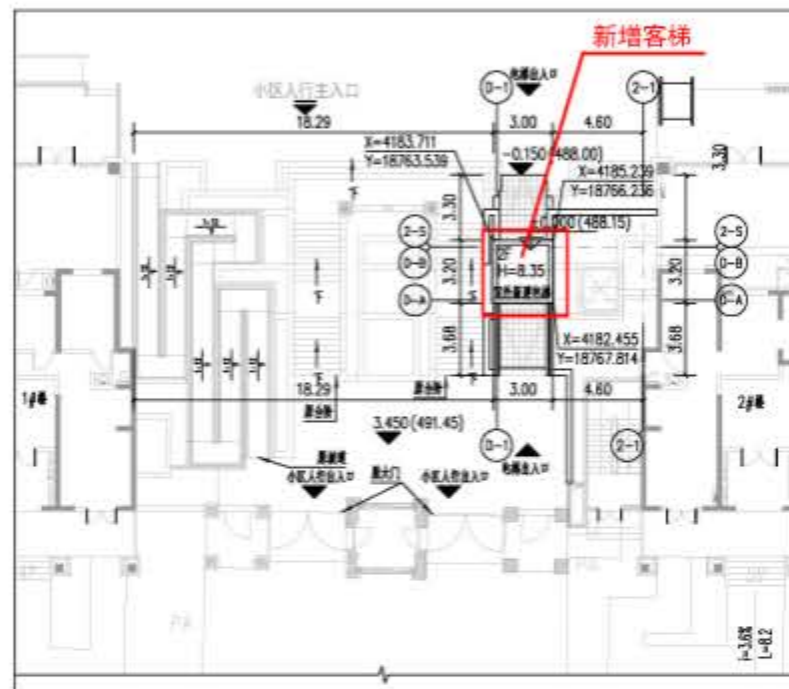
变更后平面图
