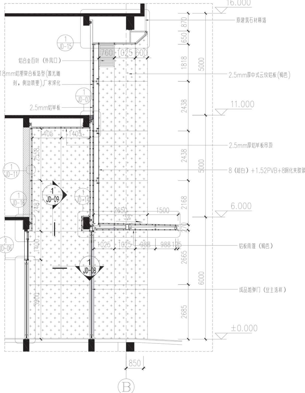
剖面图
