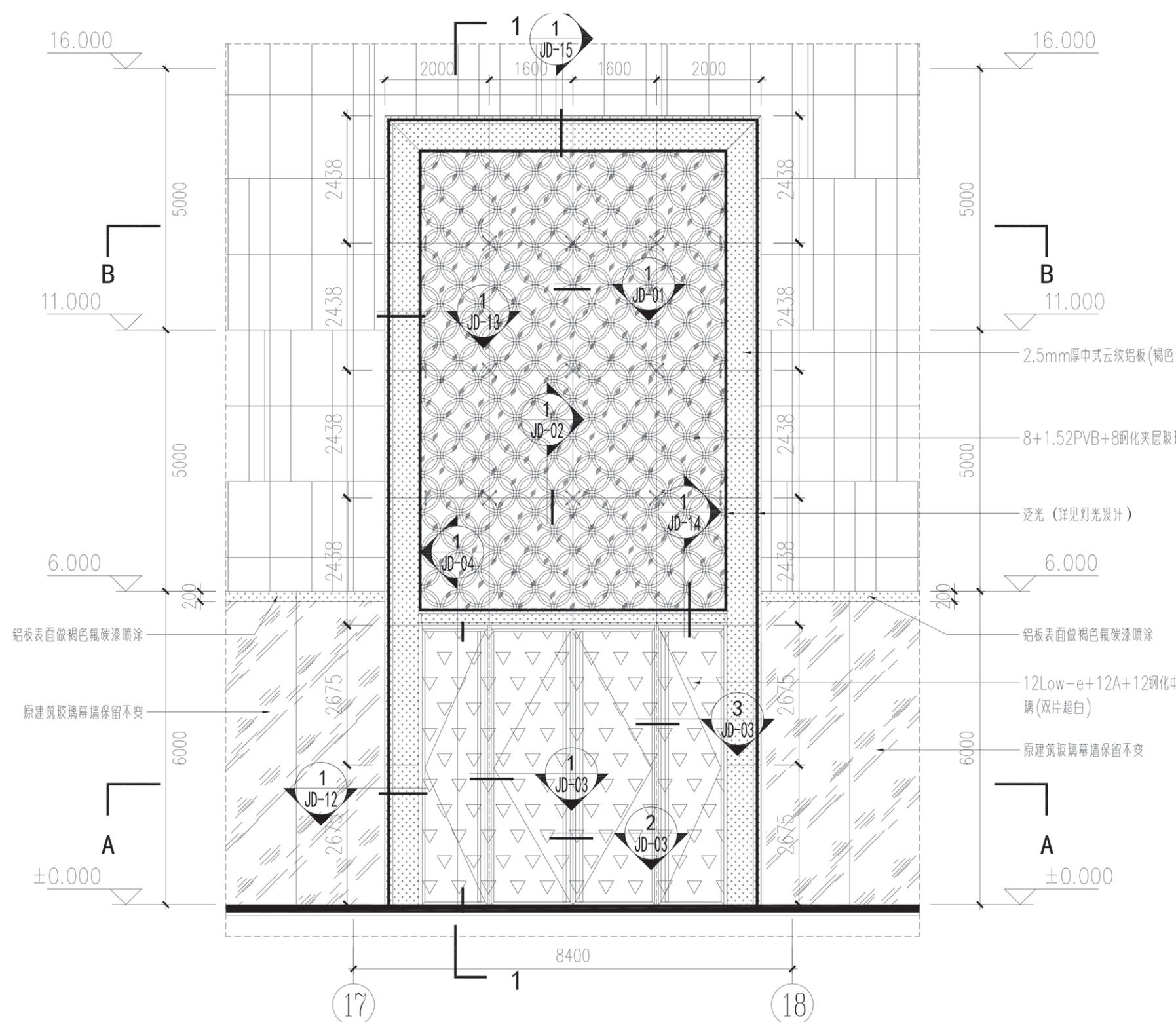
立面图
