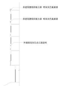
剖面图
