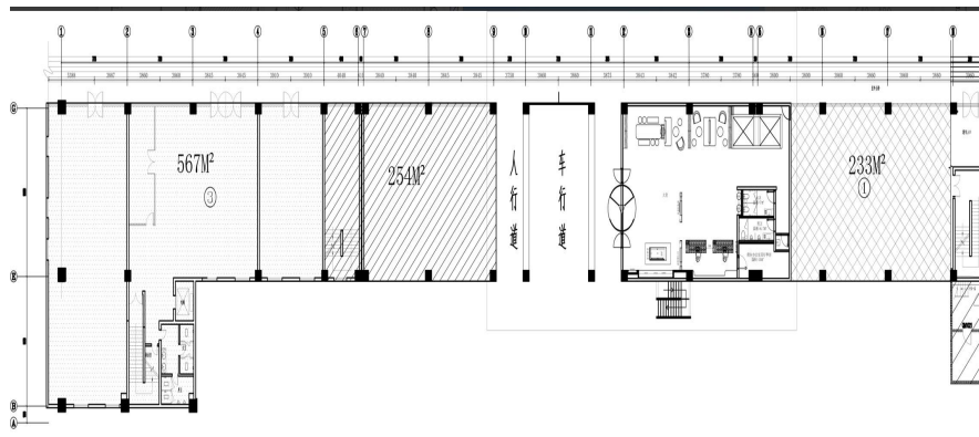
平面图
